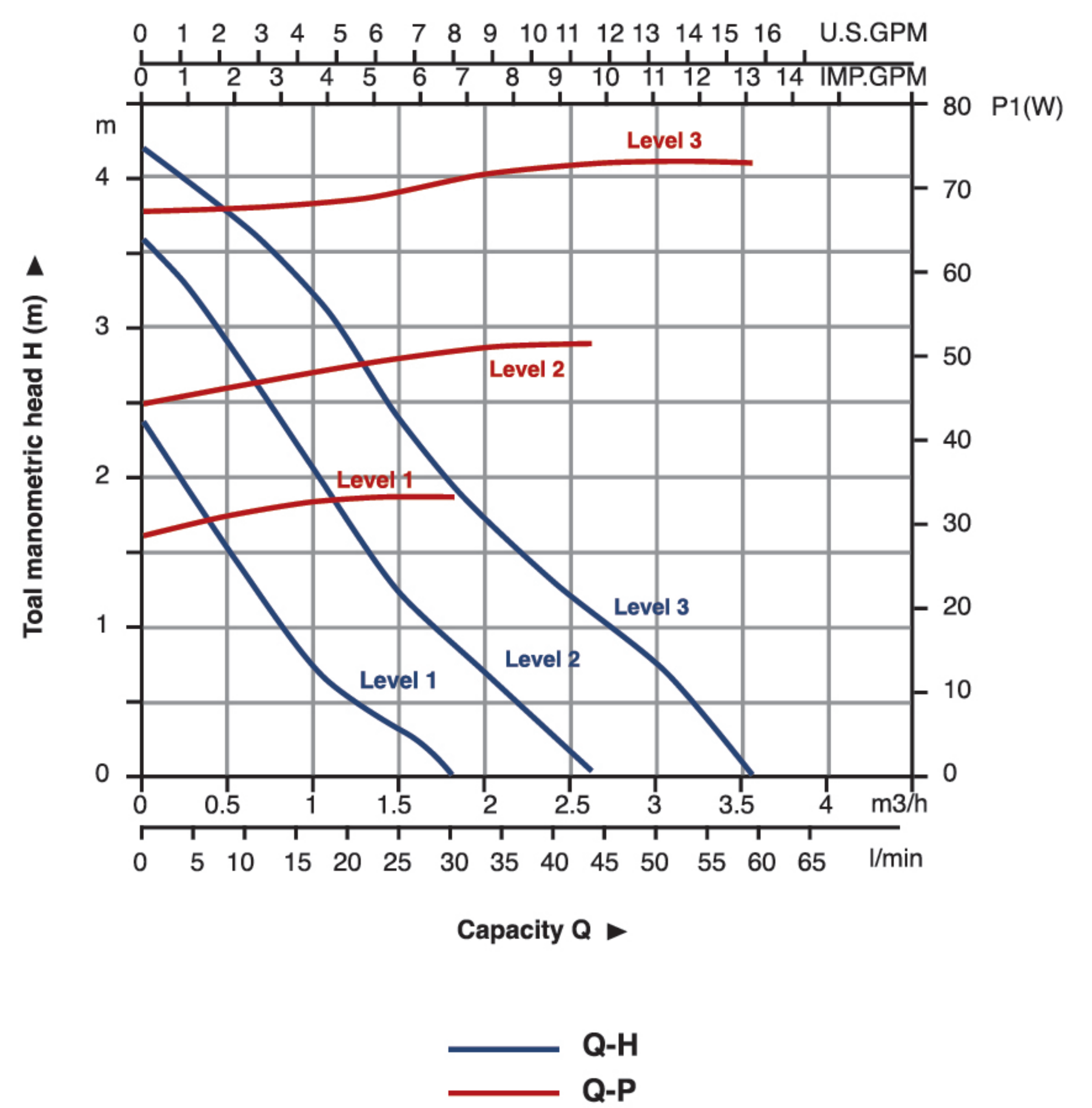
ACP 25-40/180
