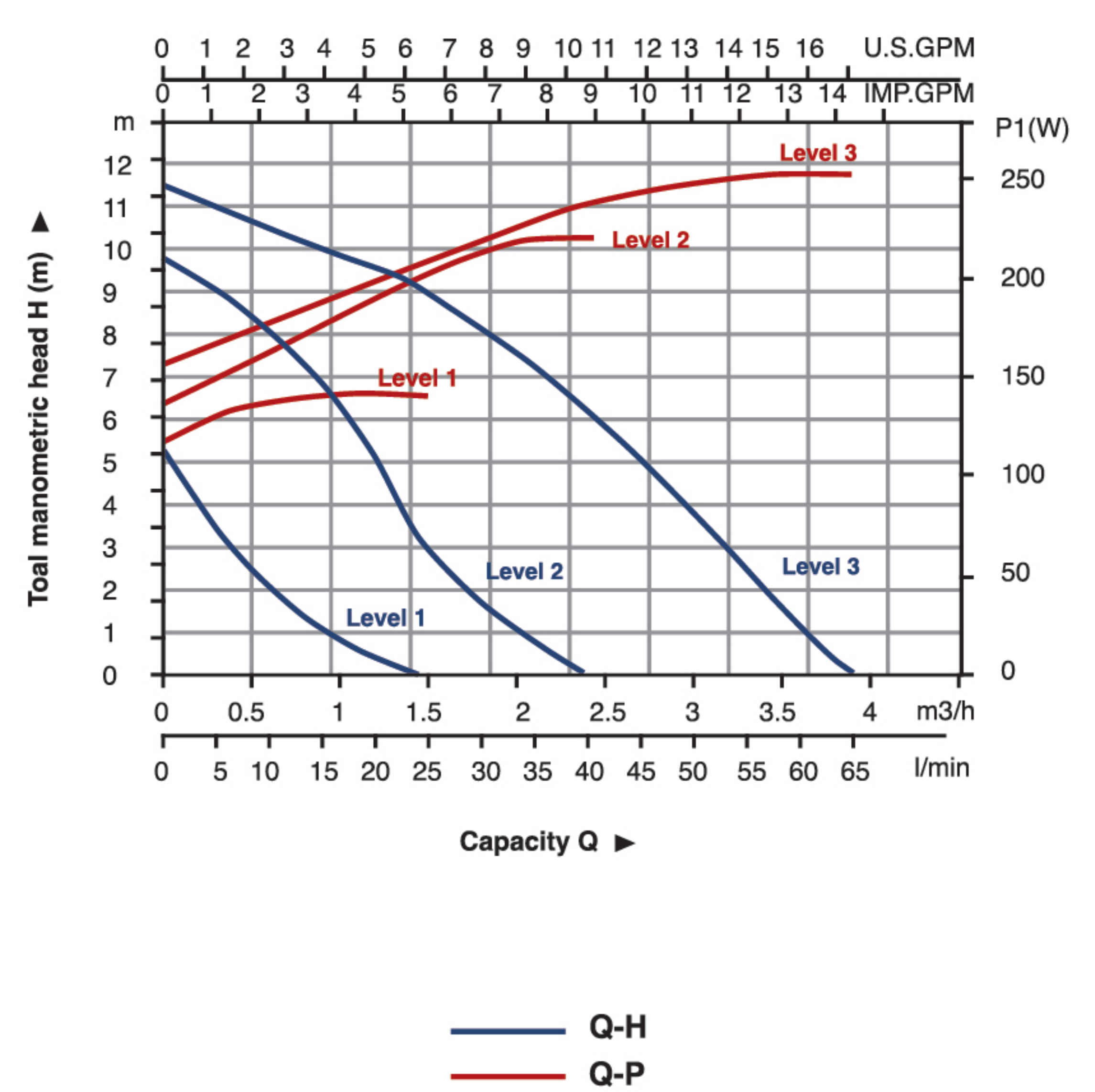
ACP 25-120/180
